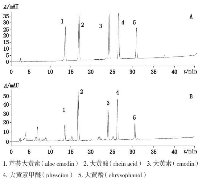
图1 混合对照品(A)和样品(B)色谱图
