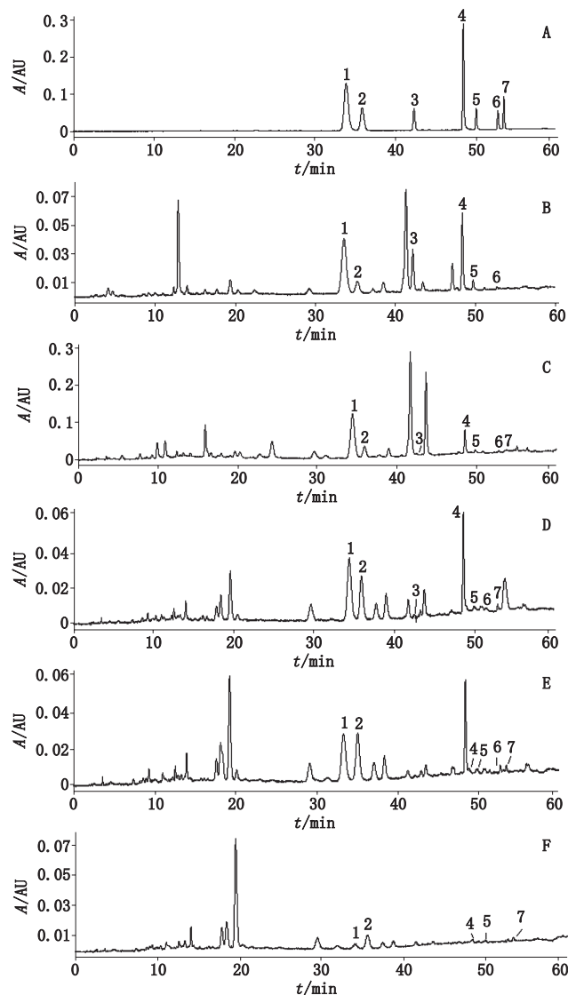
1. 金丝桃苷(hyperoside) 2. 芦丁(rutin) 3. 槲皮苷(quercitrin) 4. 槲皮素(quercetin) 5. 木犀草素(luteolin) 6. 山柰酚(kaempferol) 7. 异鼠李素(isorhamnetin) A. 混合对照品(mixed reference substances) B. 花(flowers) C. 叶(leaves) D. 嫩枝(twigs) E. 老枝(old branch) F. 根(root)
